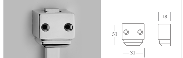
▲ RGST4 Rod End Guide/Staple
